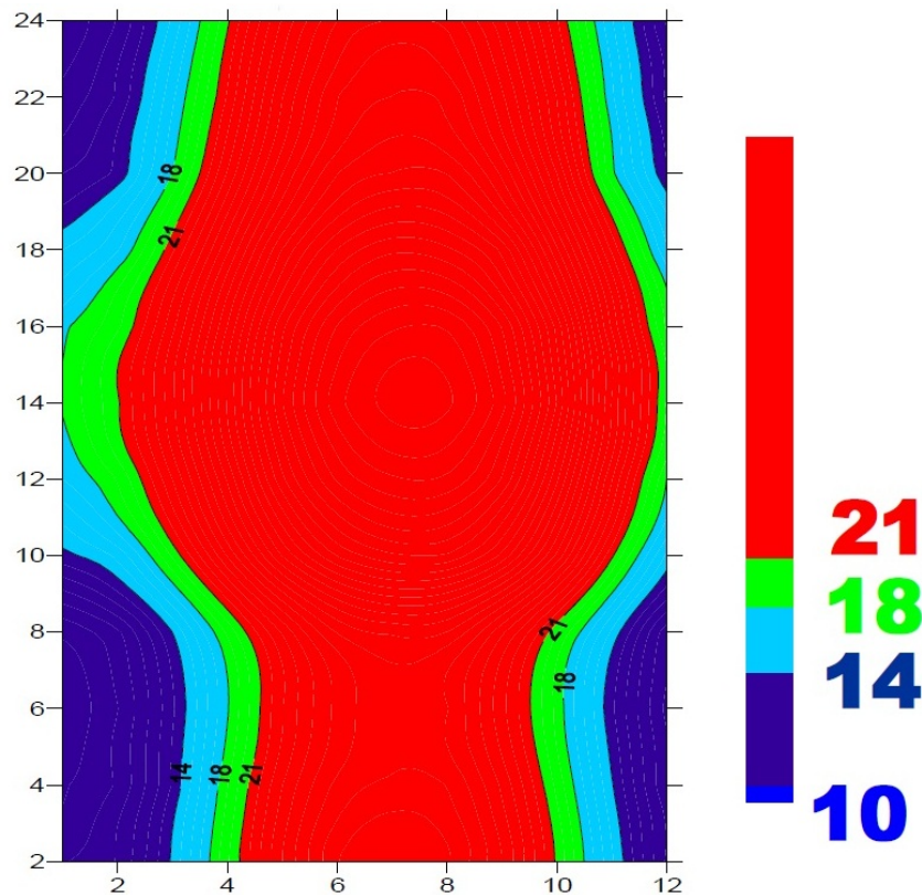
شکل ۹: نمودار هم‌دمای نیاز حرارتی داخل ساختمان شهر ماهشهر در نرم افزار Surfer (ترسیم: نگارندگان)
