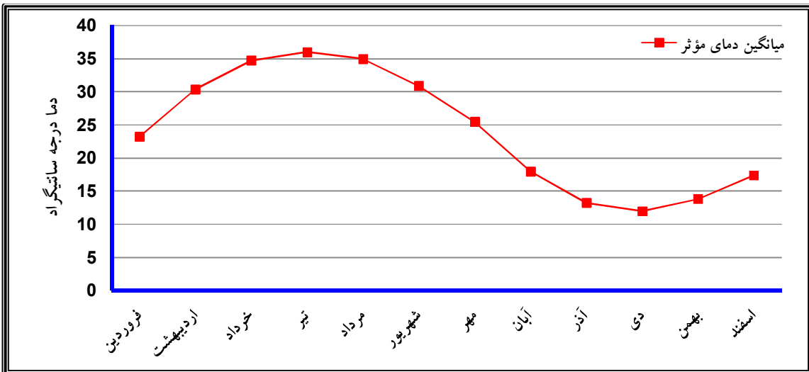
شکل شماره ۳: نمودار شاخص آسایش بیوکلیمایی دمای مؤثر شهر ماهشهر (ترسیم: نگارندگان)
