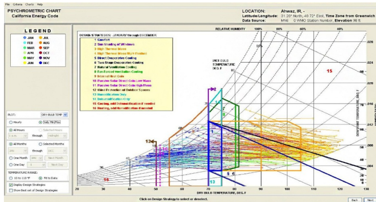
شکل ۶: نمودار زیست اقلیمی ساختمانی شهر ماهشهر بر اساس روزهای فصول سرد و گرم سال در نرم افزار Climate Consultant (ترسیم: نگارندگان)
